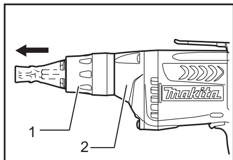
► 1. Anillo de bloqueo 2. Caja del engranaje
